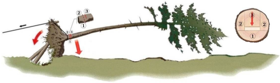
Rys.67 Kolejność i przesunięcie rzałów przy cięciu drewna o większych naprężeniach na przykładzie odcinania bryły korzeniowej wywrotów nie podpartych.
