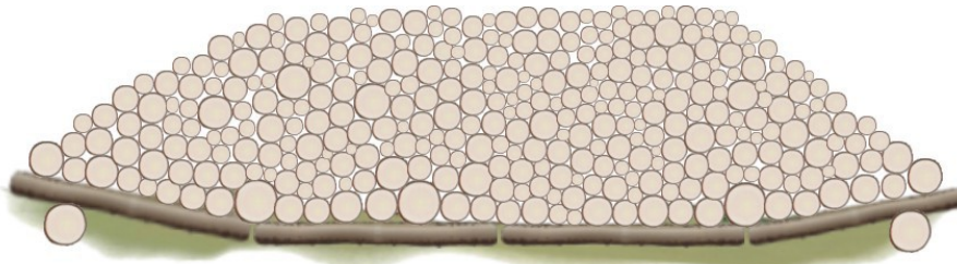
Rys.71 Przykład zabezpieczenia stosu nieregularnego.
