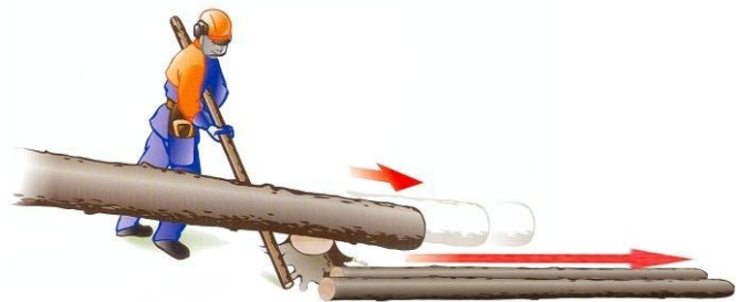
Rys.36 Ściąganie drzewa z wykorzystaniem ślizgu.
