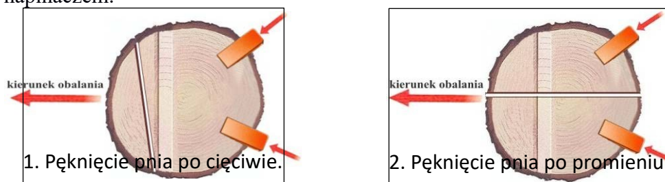
Rys.33 Wykonywanie rżazu podcinającego przy ścinie drzew z pękniętym pniem
